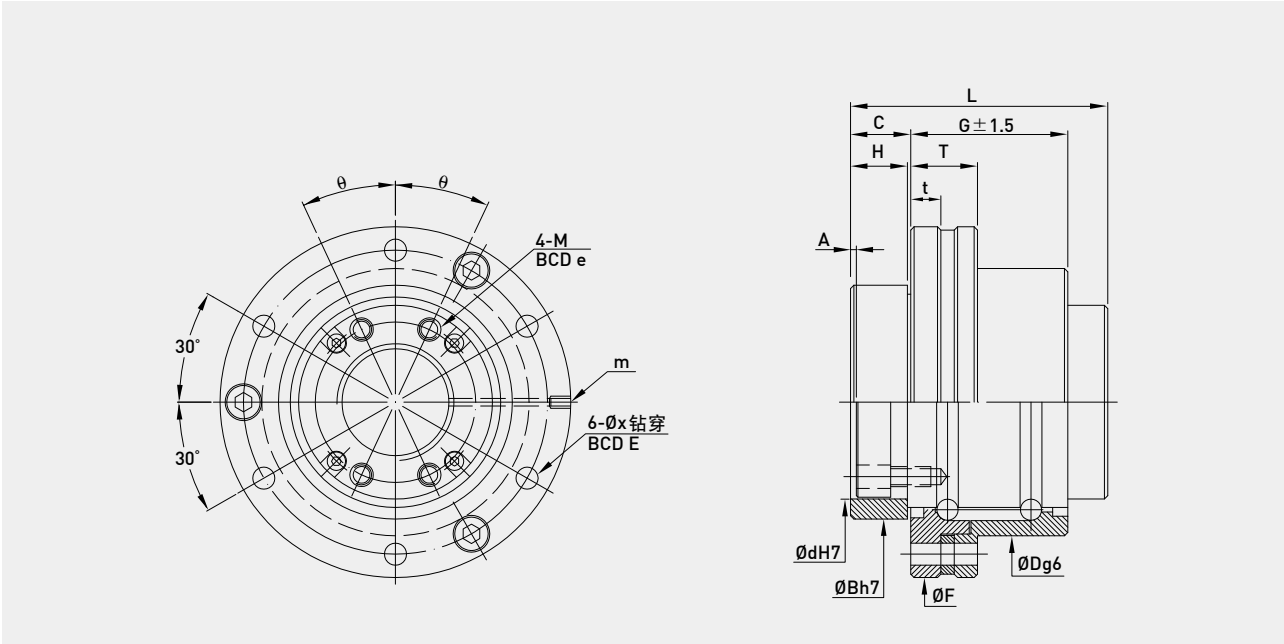
螺帽旋转式滚珠丝杠规格表
