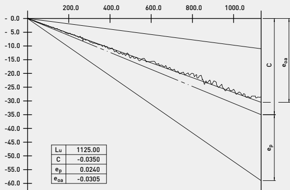
有效行程 L_u 内的平均导程偏差
