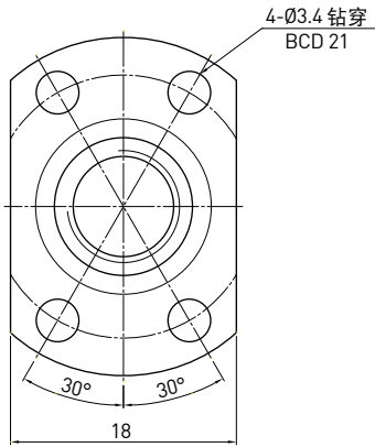
D-D 视图
