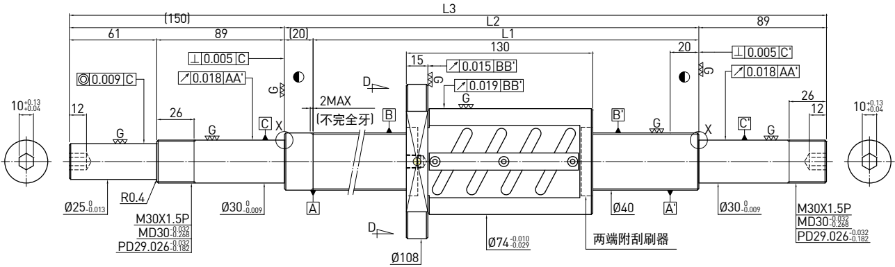
滚珠丝杠资料表
