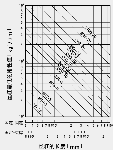
图 4.29 丝杠刚性表
