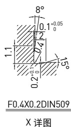
X 详图
