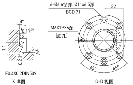
D-D 视图
