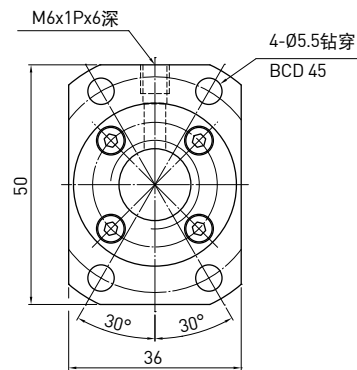
D-D 视图
