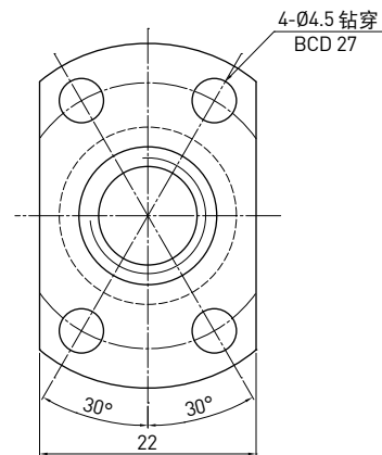
D-D 视图
