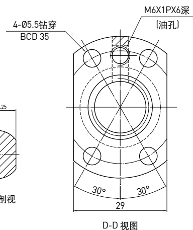
D-D 视图
