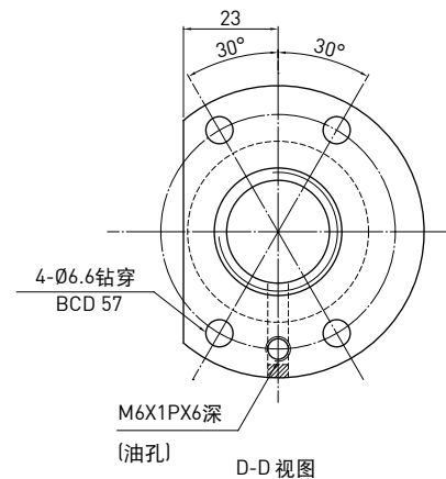
D-D 视图
