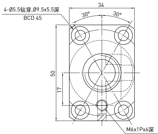
D-D 视图
